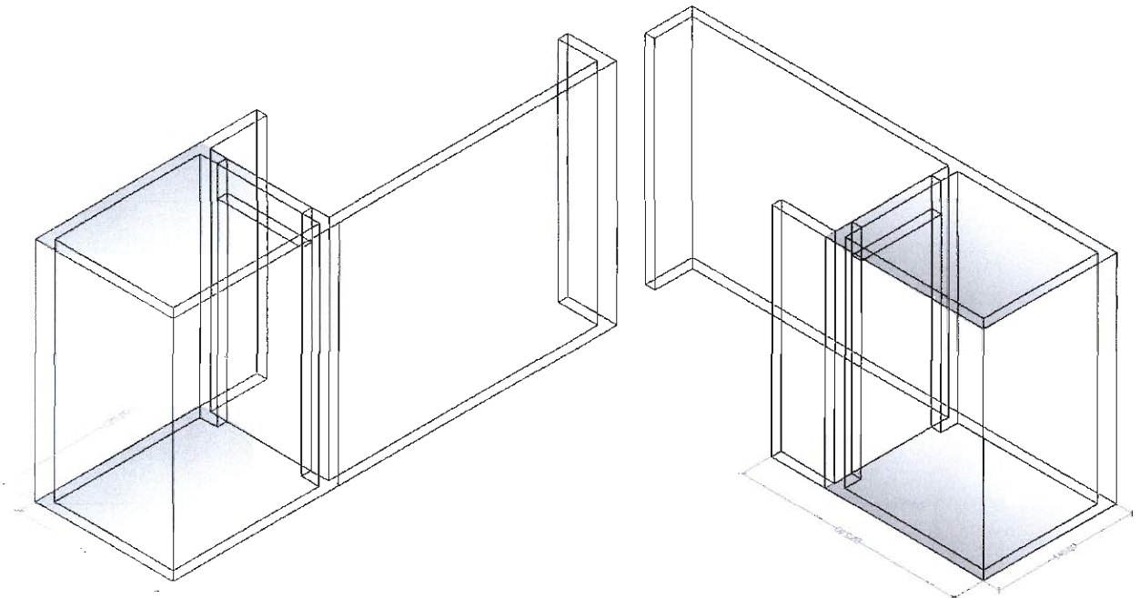
ПЛАКАР ПАРАВАН - ПРОСТОРНИ ПРИКАЗ
