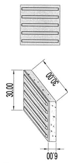
ТИП "Б" - плоча водилца за слепе и слабовиде
