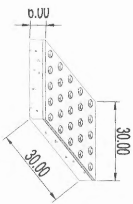
ТИП "А" - плоча улпозорена
