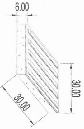
ТИП "Б" - плоча водилца за следеће и слабовидне
