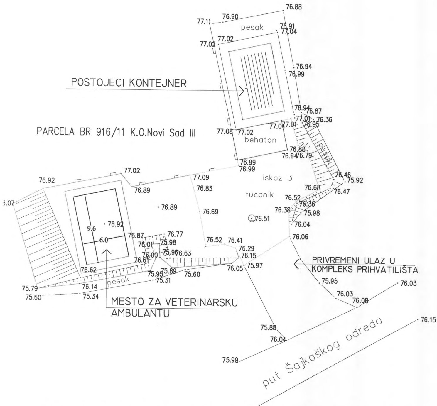
SITUACIJA - KOMPLEKS PRIHVATILISTA SA PRIVREMENIM ULAZOM
